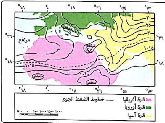
توزيع الضغط الجوي في يناير
