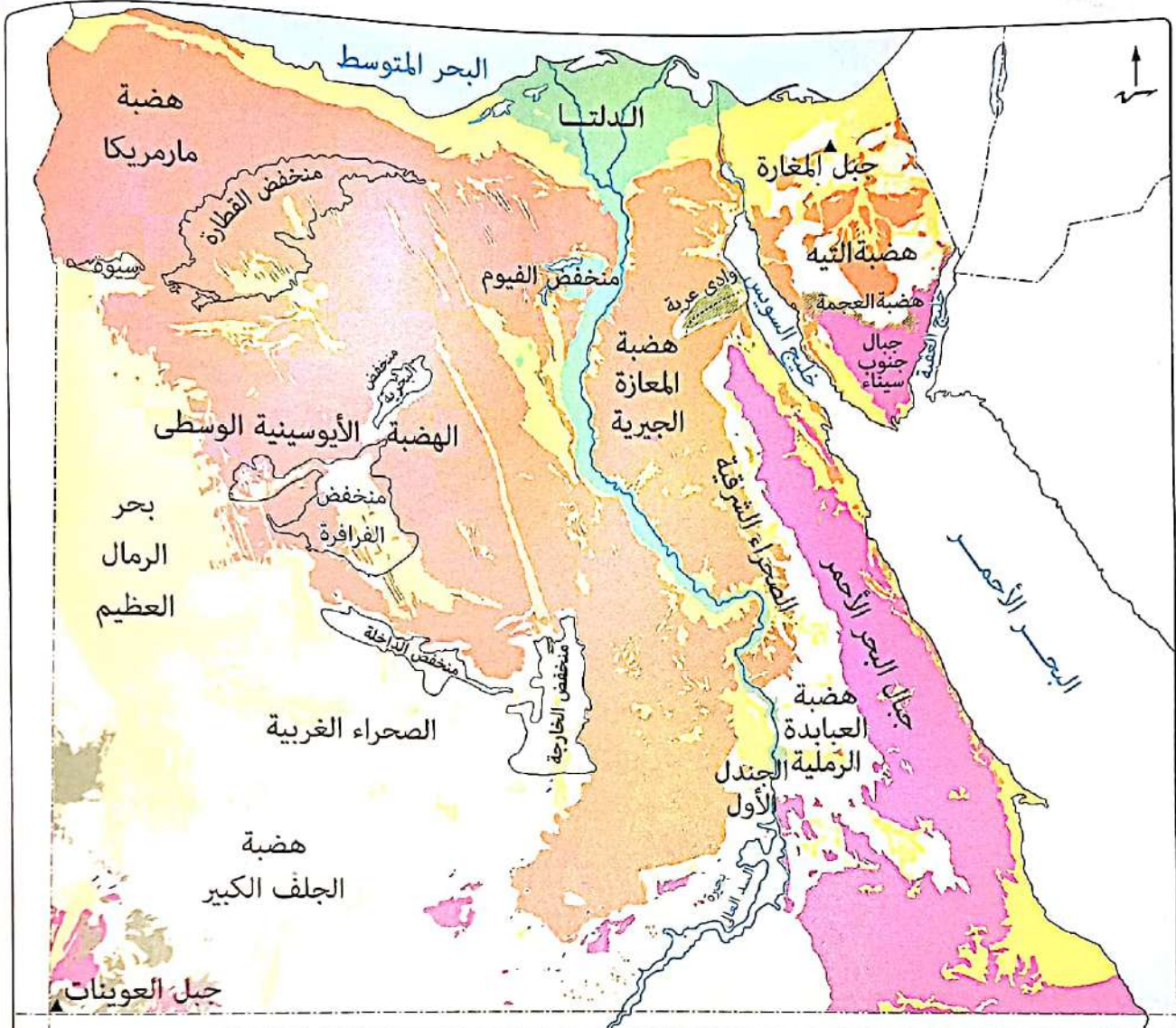
التوزيع الجغرافي لتكوينات الأزمنة الجيولوجية في مصر
