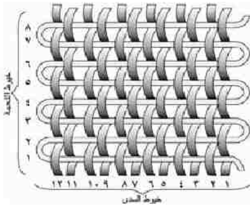
شكل (٢٩) توضح اتجاه خيوط السداة واللحمية
